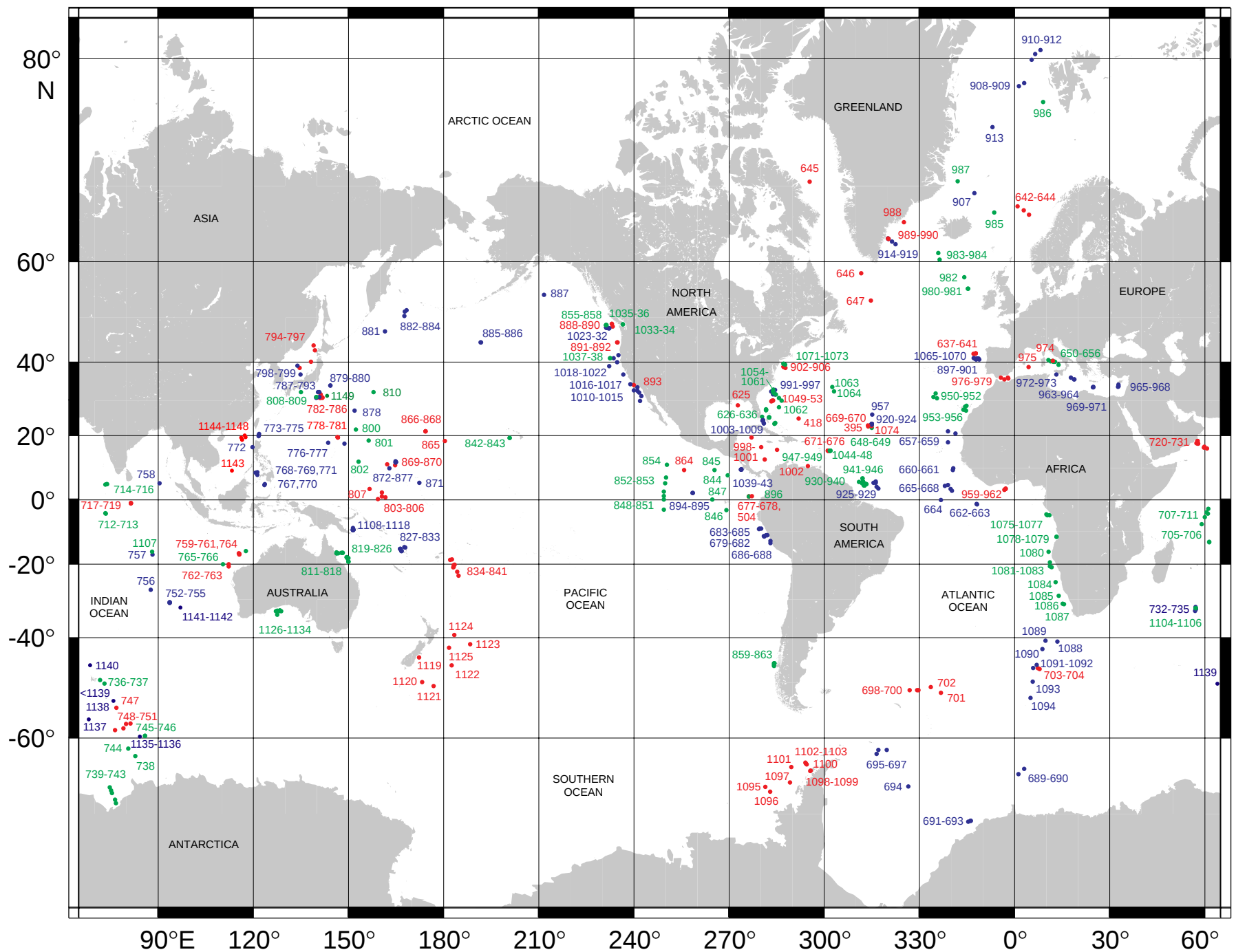
ODP Legs 100-185, Sites 625-1149
