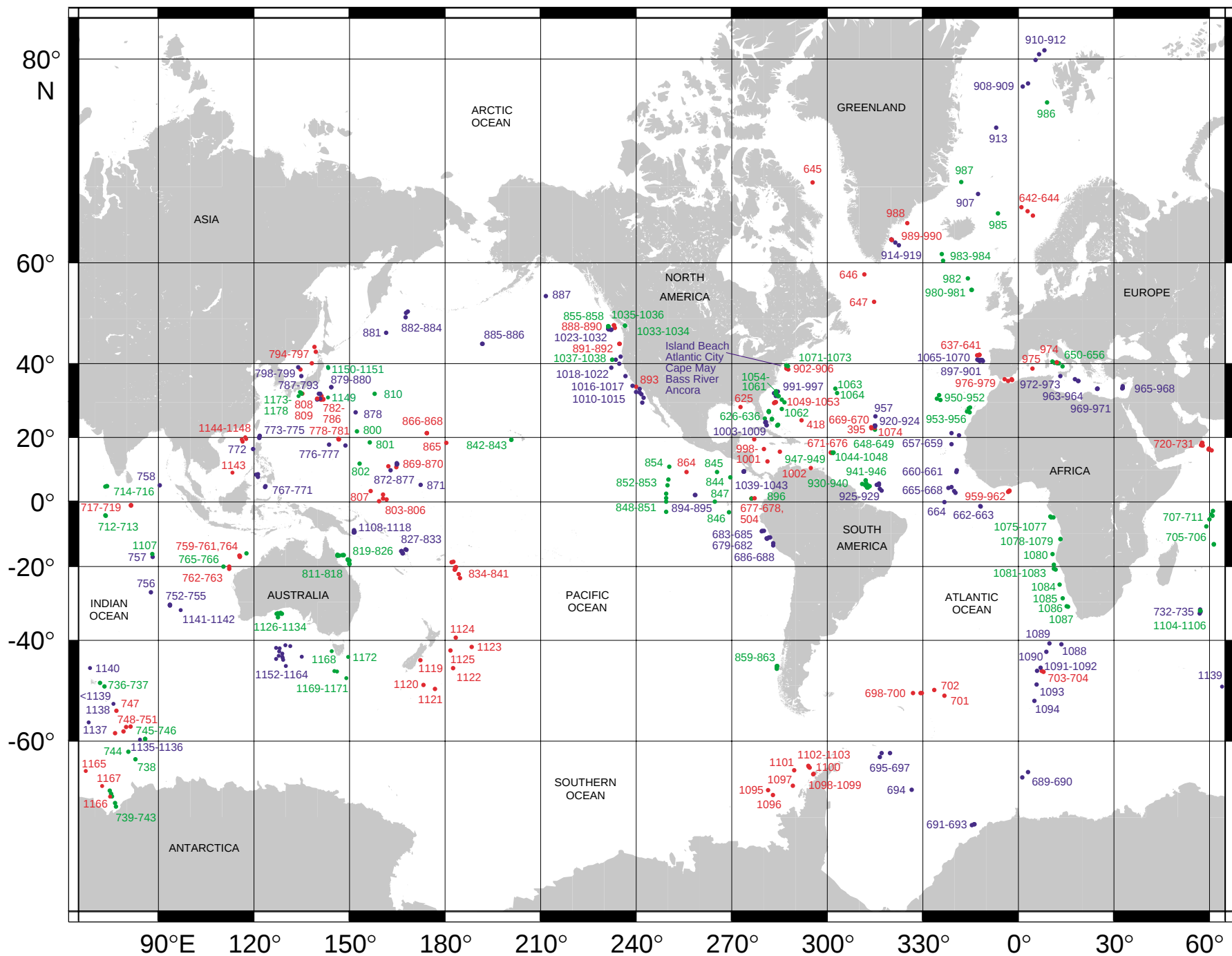
ODP Legs 100-190, Sites 625-1178
