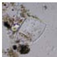
Feldspar 2
