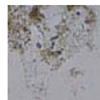
Feldspar 5
