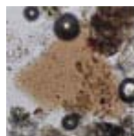
Biotite 4
