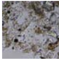
Plagioclase 3
