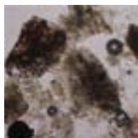
Mudstone 4
