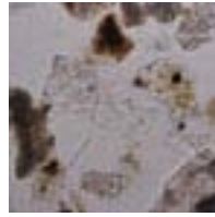
Microcline 2
