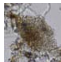
Mudstone 2
