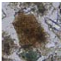
Mudstone 3
