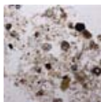
Garnet 2
