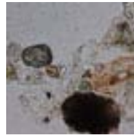
Zircon 9
