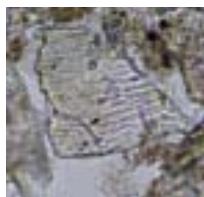
Feldspar 6
