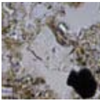
Plagioclase 1
