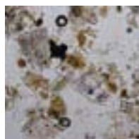
Feldspar 12
