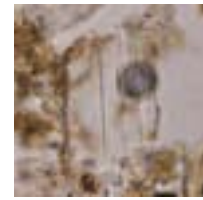
Plagioclase 5
